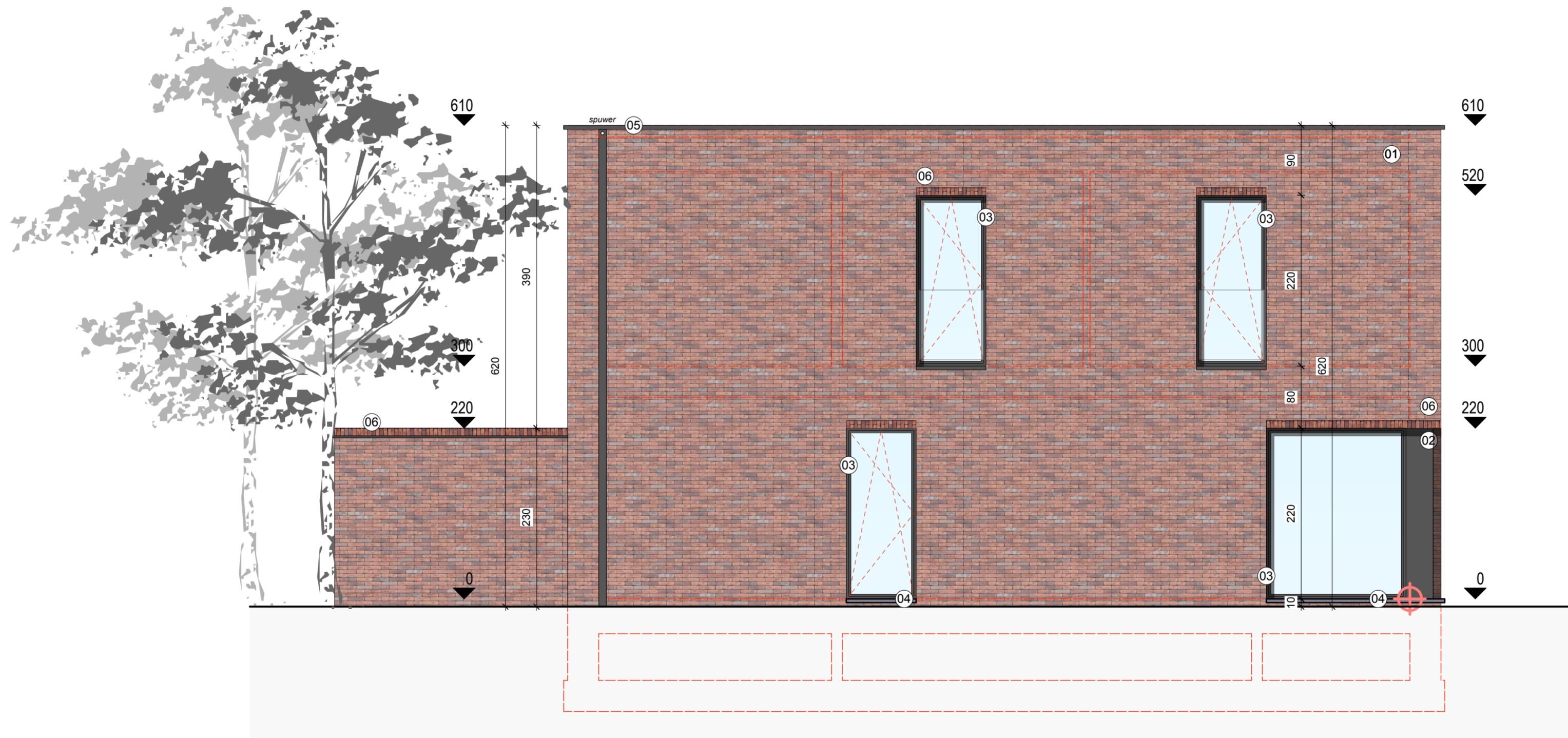
LINKER ZIJGEVEL 1/50
